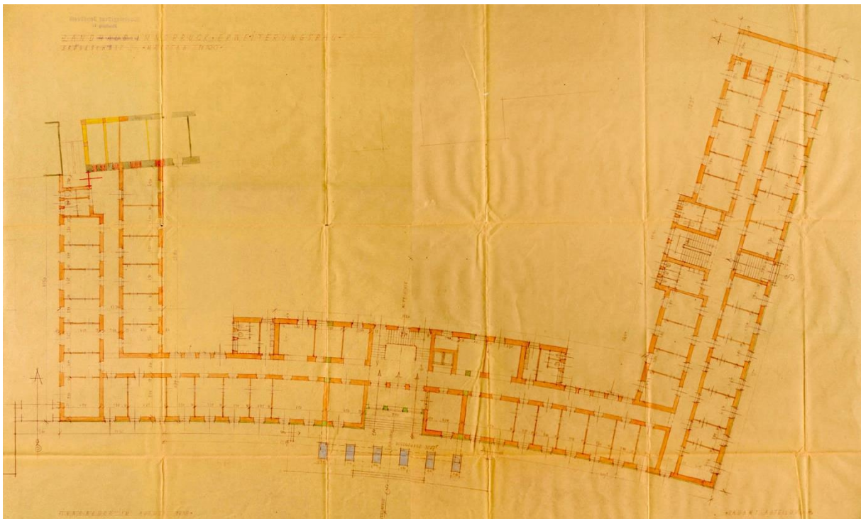
Abb. 14, Walter und Ewald Guth, Landhaus-Erweiterungsbau, Wettbewerbseinreichung, Grundriss des Erdgeschosses. Die Brüder Guth gehen von 6 Pfeilern der vorgesetzten Eingangshalle aus und planen ein zentrales Treppenhaus. Die Südflügel werden zum Teil von Räumen zu beiden Seiten gesäumt. Der rückwärtige Wirtschaftstrakt fehlt (TLA, Plansammlung, Landesbaudirektionspläne, Innsbruck, Landhaus T.39-17).
