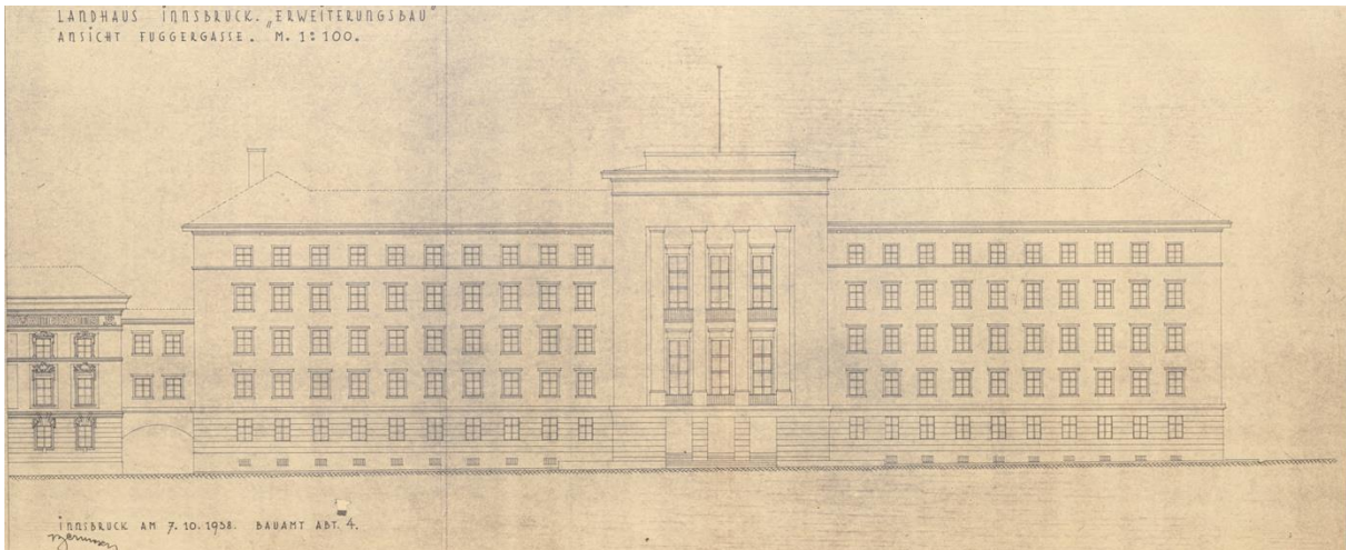
Abb. 19, Albert Bermoser, Überarbeitung der Südfassade, Erweiterung um eine weitere Fensterachse an beiden Seitenflügeln, Einfügen neoklassizistischer Elemente wie Abschlüsse der Pilaster, eines Rustikasockels und fassadengliedernder Gurtgesimse (Registratur der Liegenschaftsverwaltung).
