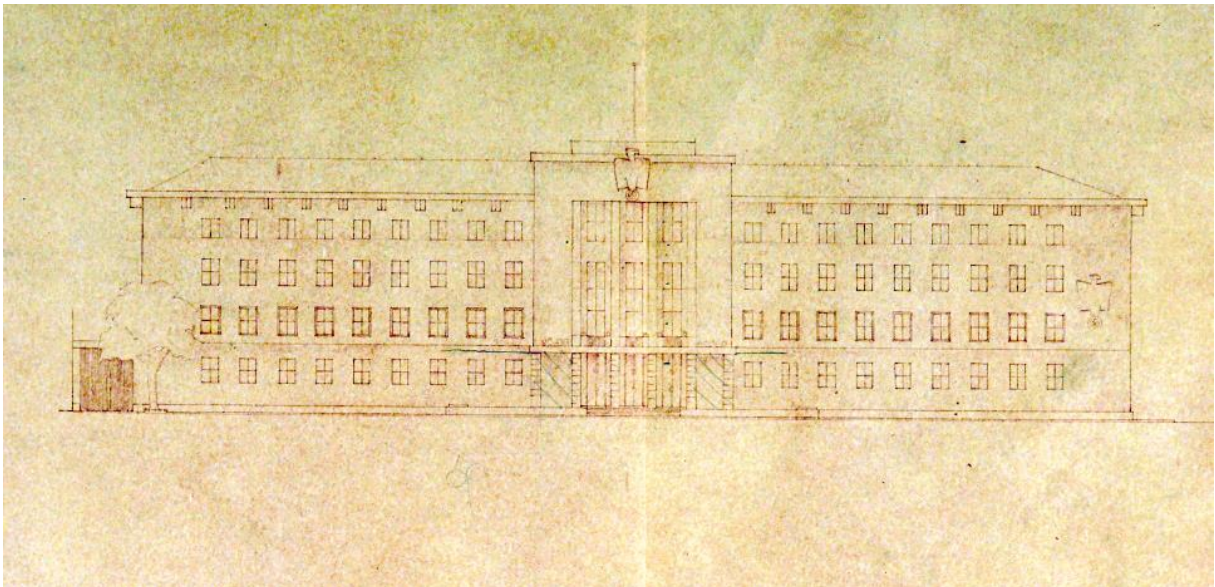
Abb. 8, Walter und Ewald Guth, Wettbewerbsbeitrag, Landhaus-Erweiterungsbau, Ansicht Südfassade, August 1938. Der Entwurf sieht 4 Geschosse und 9 Fensterachsen an den beiden Seitenflügeln vor. Der erhöhte Mittelrisalit ist betont nüchtern gestaltet und vertikal und horizontal akzentuiert (Registratur der Liegenschaftsverwaltung).
